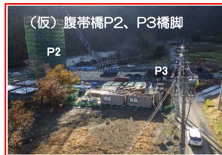
(仮)腹帯橋P2、P3橋脚 P2橋脚は柱部の全長約30mのうち半分が完了しています。P3橋脚は底盤部の埋戻しを行っています。
